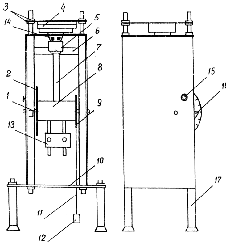
Схема стенда "ПРЯМОЙ УДАР":
