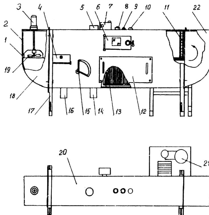
Схема стенда "ТЕПЛОВОЙ - ДЫМОВОЙ КАНАЛ":
