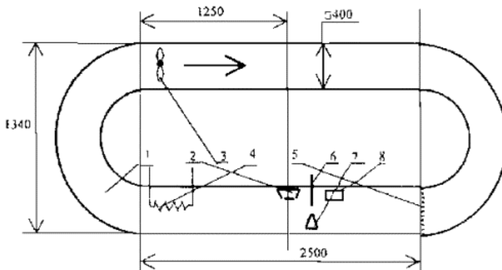
Схема измерительной камеры:
