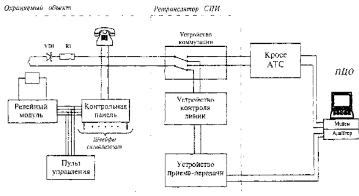
Рисунок 1 - Реализация КСЦО с использованием релейного модуля
