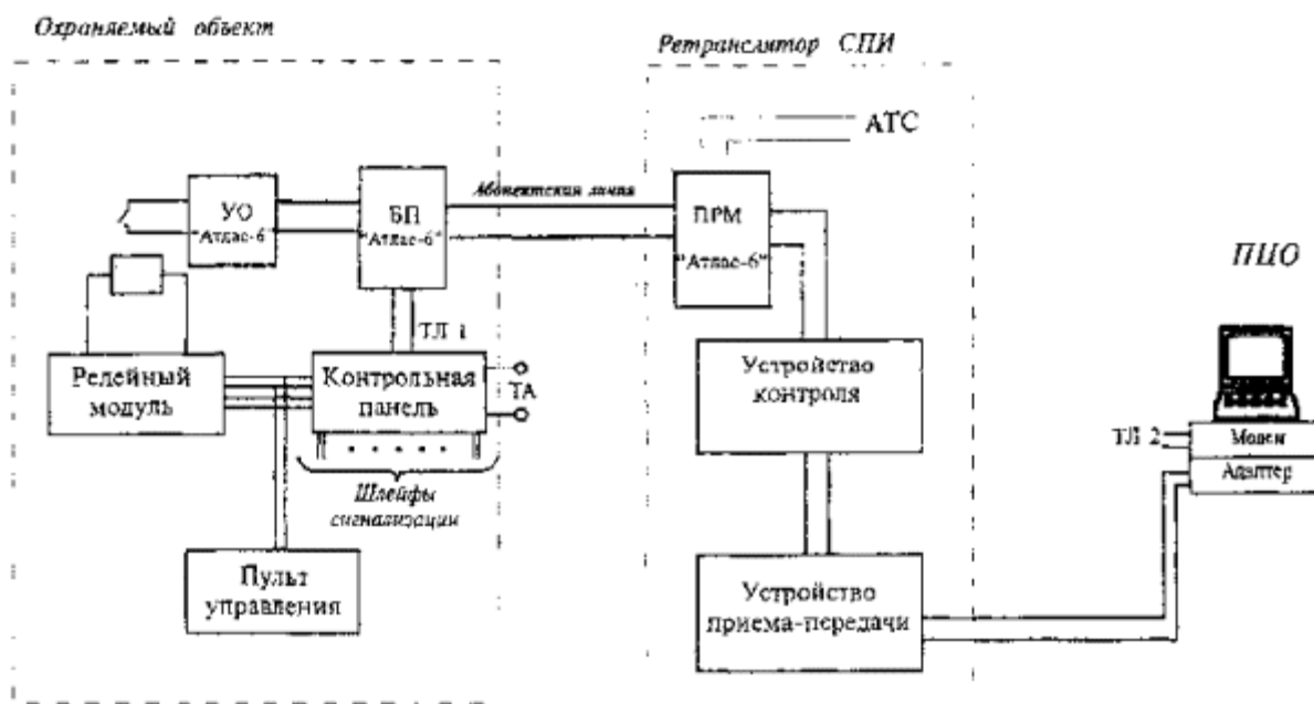
Рисунок 3 - Реализация КСЦО с использованием релейного модуля и аппаратуры "Атлас-6"
